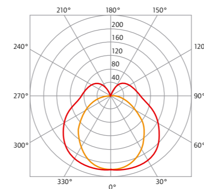
LICHTVERTEILUNGSKURVE 12 Watt (SL14a.12CW.O.S0W4)
