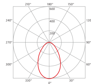
LICHTVERTEILUNGSKURVE 15 Watt (6151nD.1540.A0.81)
