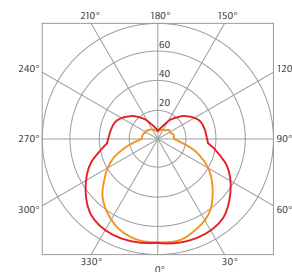
LICHTVERTEILUNGSKURVE 21 Watt (5612.2140.TO.80)
