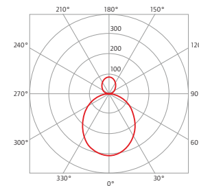
LICHTVERTEILUNGSKURVE 29 Watt (2842.2940.OPl.80)
