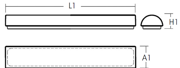
Bauform 5611
